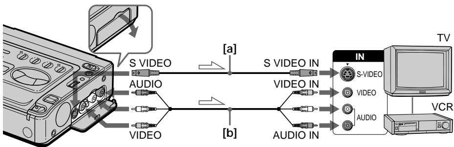
➤ : Signalfuß / Direzione del segnale
